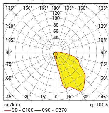
Полярная диаграмма
